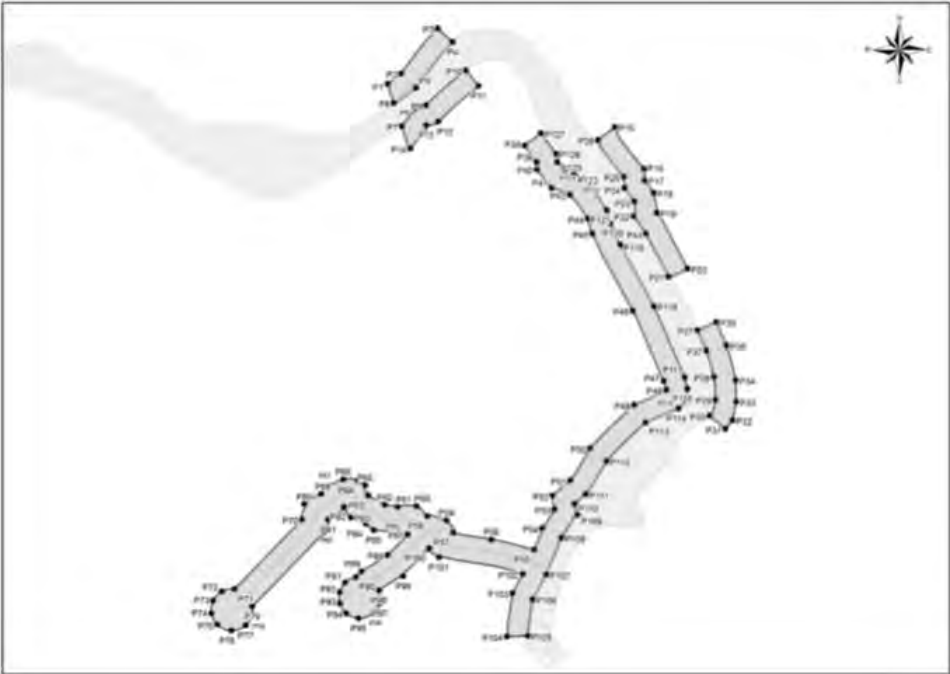
Croqui da Área de Preservação Permanente onde ocorrerá a intervenção Coordenadas de Referência UTM DATUM SIRGAS 2000
